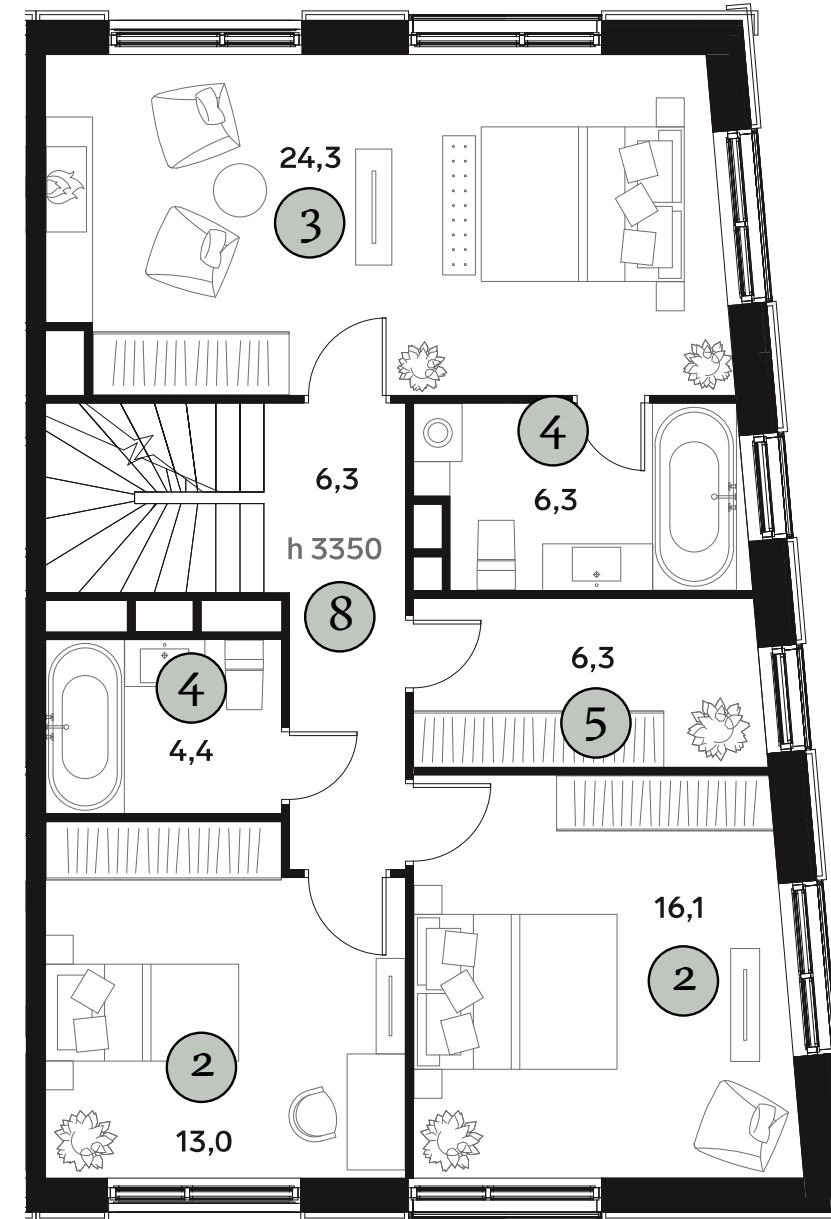
2-й этаж
